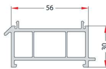
30 x 56 EXTENDER PROFILE 30 x 56 YÜKSELTME PROFİLİ EN 114 HIGHLINE
