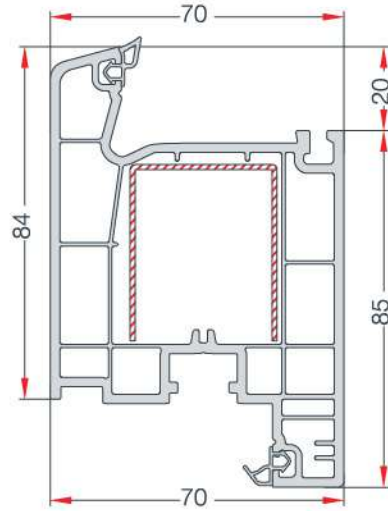
DOOR SASH PROFILE KAPI KANAT PROFİLİ EN 213
