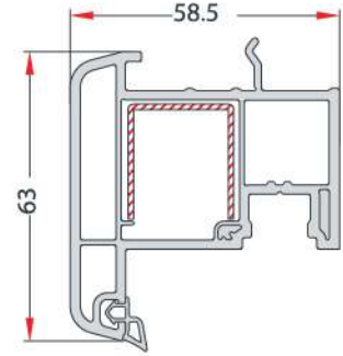
MOVABLE MULLION PROFILE HAREKETLİ ORTA KAYIT PROFİLİ EN 25
