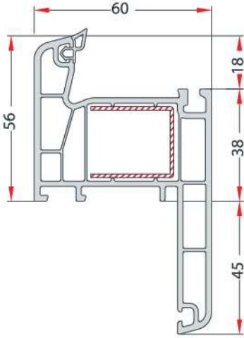
FRAME PROFILE KASA PROFİLİ EN 81
