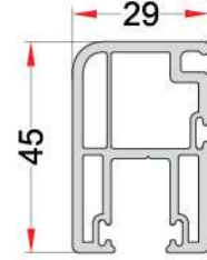
FLY SCREEN PROFILE SİNEKLİK PROFİLİ EN 34
