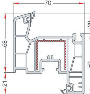
WINDOW SASH PROFILE PENCERE KANAT PROFİLİ EN 18
