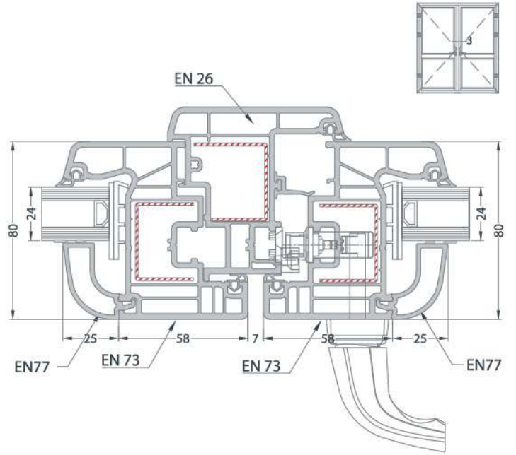
MOVABLE MULLION - WINDOW SASH INSTALLATION HAREKETLİ ORTA KAYIT - PENCERE KANAT UYGULAMASI
