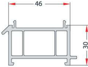
30 x 46 EXTENDER PROFILE 30 x 46 YÜKSELTME PROFİLİ EN 113 KLASLINE
