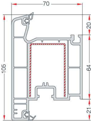
OUTWARD OPENING DOOR SASH PROFILE DIŞA AÇILIM KAPI KANAT PROFİLİ EN 22
