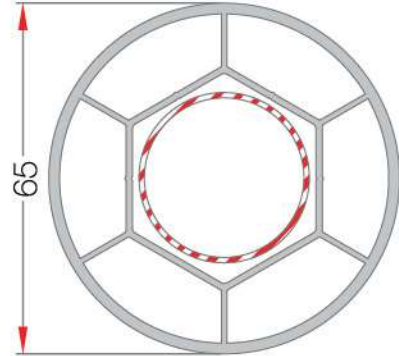
Ø65 PIPE PROFILE Ø65 BORU PROFİLİ EN 28
