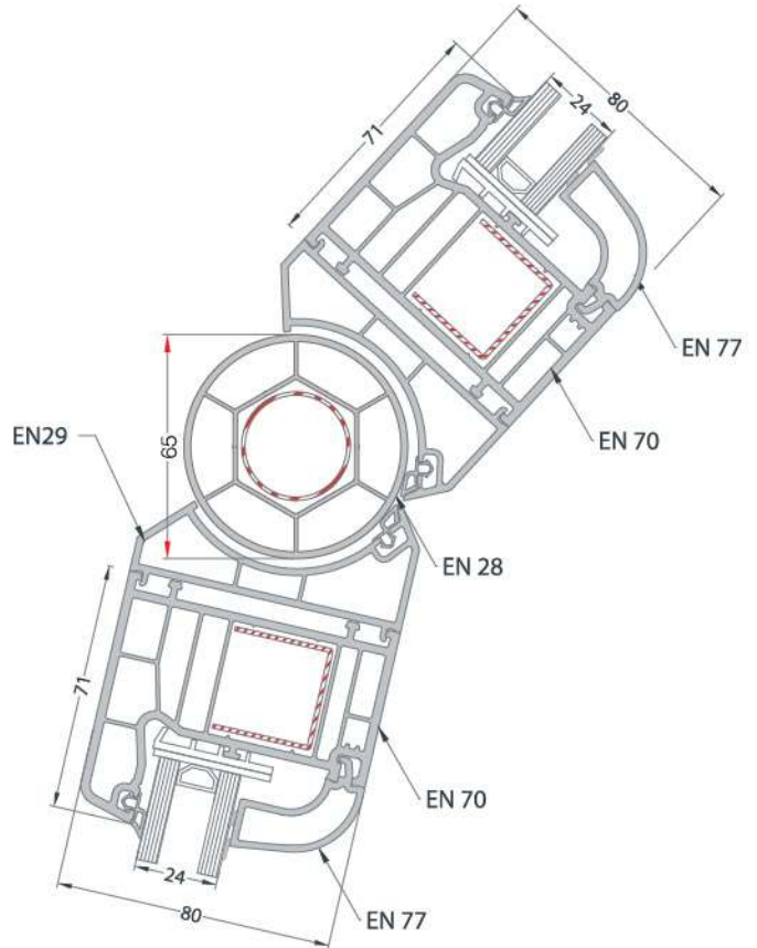
CORNER ADAPTER INSTALLATION AÇILI DÖNÜŞ ADAPTÖRÜ UYGULAMASI
