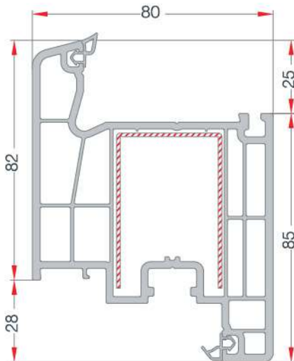
DOOR SASH PROFILE KAPI KANAT PROFİLİ EN 74
