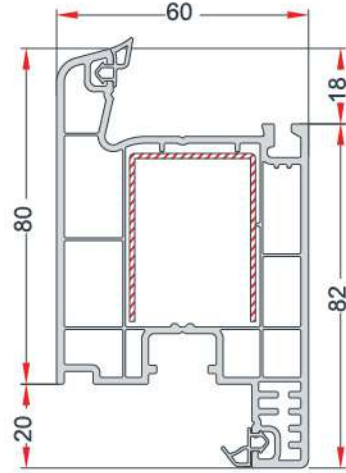
DOOR SASH PROFILE KAPI KANAT PROFİLİ EN 842
