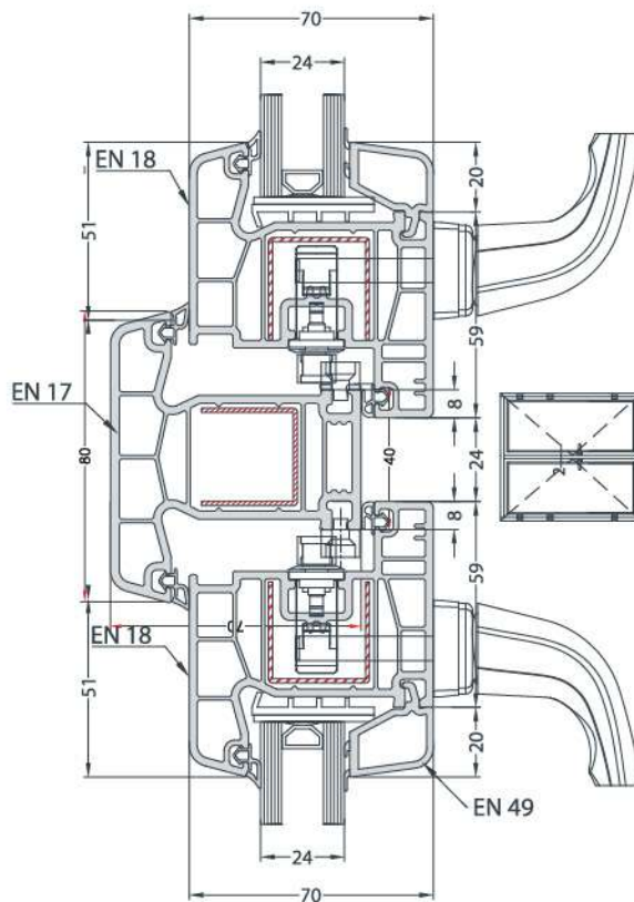
MULLION - WINDOW SASH INSTALLATION ORTA KAYIT - PENCERE KANAT UYGULAMASI
