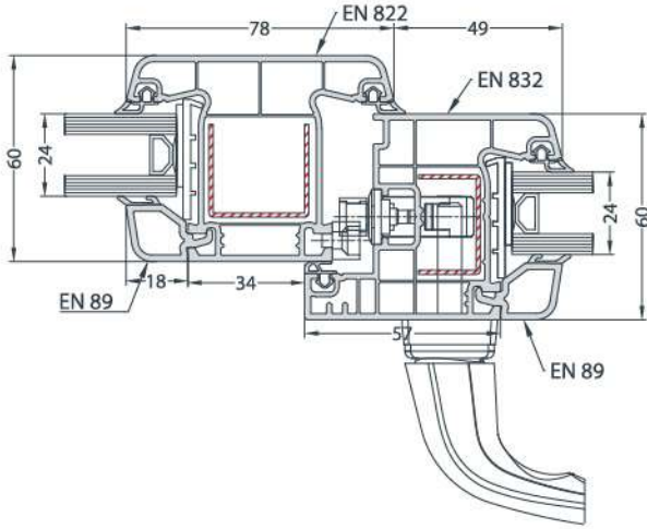
MULLION - WINDOW SASH INSTALLATION ORTA KAYIT PENCERE KANAT UYGULAMASI
