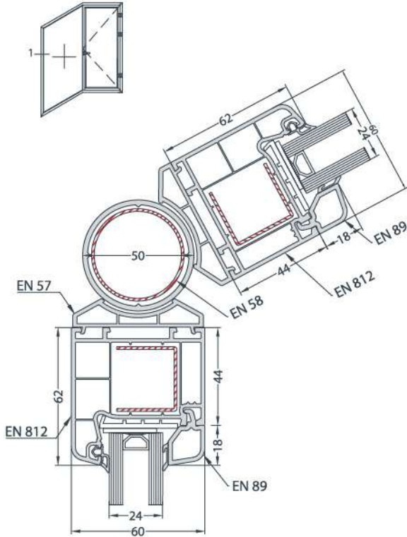
MULLION - WINDOW SASH INSTALLATION ORTA KAYIT PENCERE KANAT UYGULAMASI
