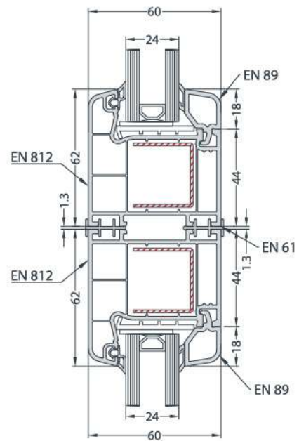
UNIVERSAL COUPLING PROFILE INSTALLATION ÜNİVERSAL BAĞ PROFİLİ UYGULAMASI
