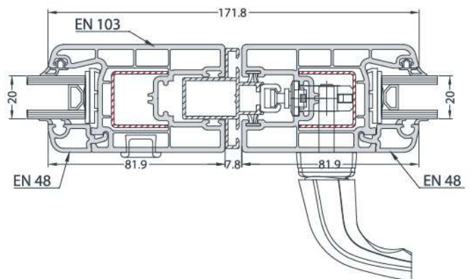
SLIDING ALUMINIUM CONNECTOR INSTALLATION SÜRME ALÜMİNYUM BİRLEŞTİRME ADAPTÖR UYGULAMASI
