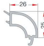
32-mm TRIPLE GLAZING BEAD 32 mm ÜÇLÜ CAM ÇİTASI EN 78
