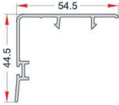
SLIDING LOCK ADAPTER PROFILE SÜRME KİLİT ADAPTÖR PROFİLİ EN 99
