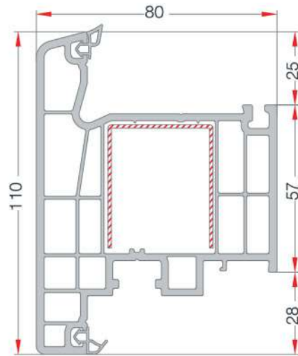
OUTWARD OPENING DOOR SASH PROFILE DIŞA AÇILIM KAPI KANAT PROFİLİ EN 75
