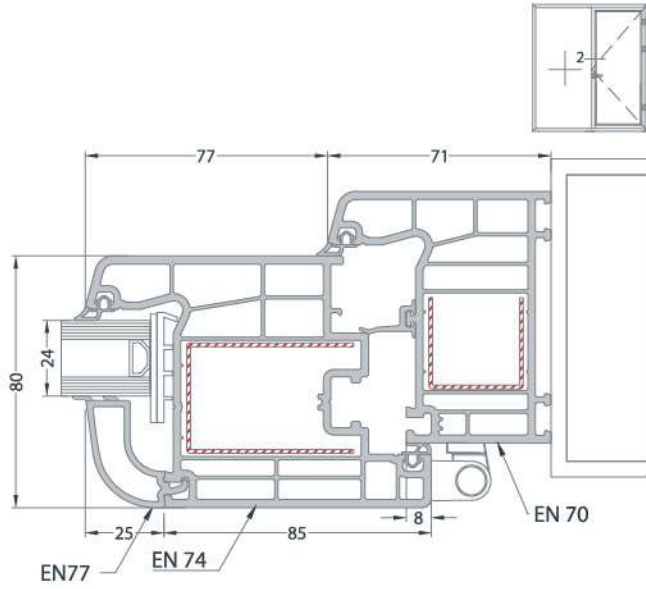
FRAME - DOOR SASH INSTALLATION KASA - KAPI KANAT UYGULAMASI
