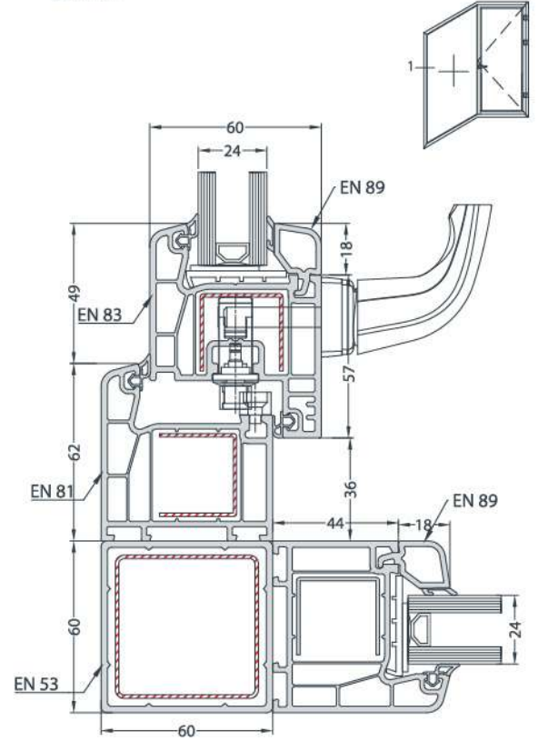
BOX PROFILE INSTALLATION KUTU PROFİLİ UYGULAMASI
