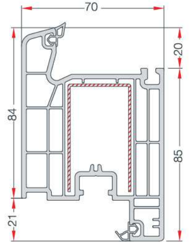
DOOR SASH PROFILE KAPI KANAT PROFİLİ EN 21
