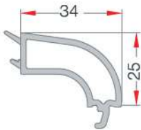
24-mm DOUBLE GLAZING BEAD 24 mm ÇİFT CAM ÇİTASI EN 77
