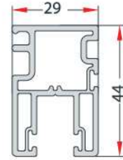
SLIDING FLY SCREEN SASH PROFILE SÜRME SİNEKLİK KANAT PROFİLİ EN 341
