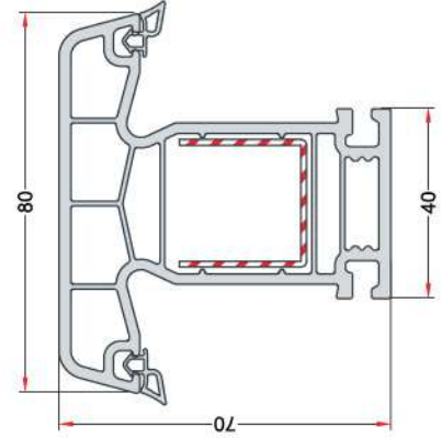
MULLION PROFILE ORTA KAYIT PROFİLİ EN 173
