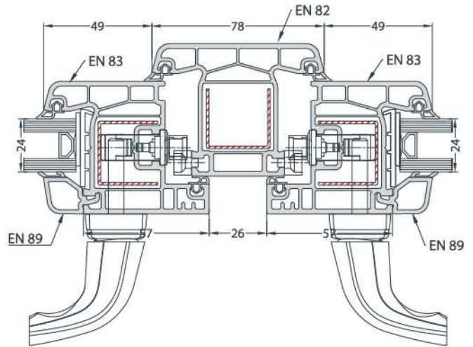
MULLION - WINDOW SASH INSTALLATION ORTA KAYIT - PENCERE KANAT UYGULAMASI
