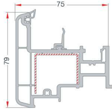
MOVABLE MULLION PROFILE HAREKETLİ ORTA KAYIT PROFİLİ EN 26
