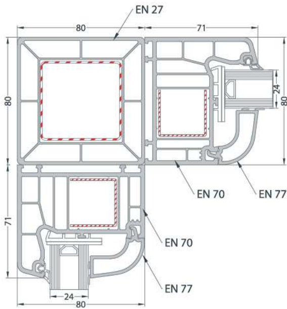
BOX PROFILE INSTALLATION KUTU PROFİLİ UYGULAMASI
