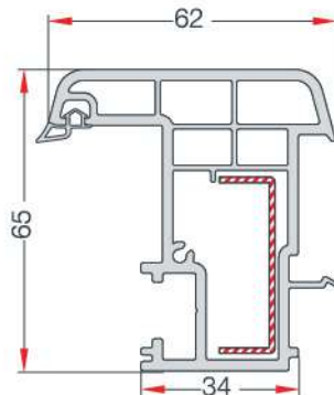
MOVABLE MULLION PROFILE HAREKETLİ ORTA KAYIT PROFİLİ EN 24
