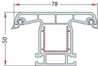
SLIDING MULLION PROFILE SÜRME ORTA KAYIT PROFİLİ EN 96
