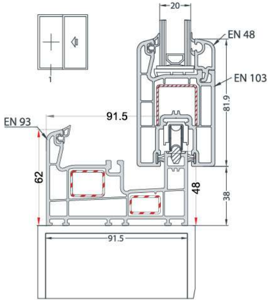
SINGLE RAILED SLIDING FRAME - SLIDING SASH INSTALLATION SÜRME TEK RAYLI KASA - SÜRME KANAT UYGULAMASI
