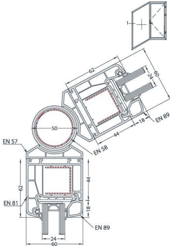
CORNER ADAPTER INSTALLATION KÖŞE DÖNÜŞ ADAPTÖRÜ UYGULAMASI
