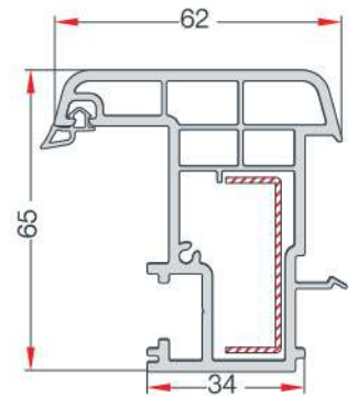
DOOR SASH PROFILE KAPI KANAT PROFİLİ EN 21
