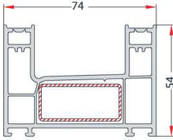
FRAME PROFILE KASA PROFİLİ EN 91
