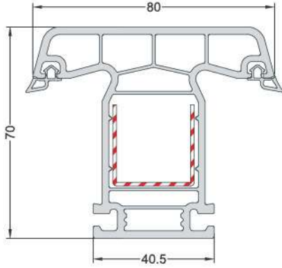
MULLION PROFILE ORTA KAYIT PROFİLİ EN 17
