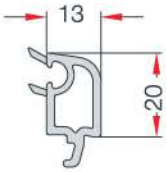
32-mm TRIPLE GLAZING BEAD 32 mm ÜÇLÜ CAM ÇİTASI EN 48
