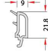
24-mm DOUBLE GLAZING BEAD 24 mm ÇİFT CAM ÇİTASI EN 109
