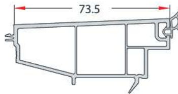
THRESHOLD CLOSING PROFILE EŞİK KAPAMA PROFİLİ EN 344
