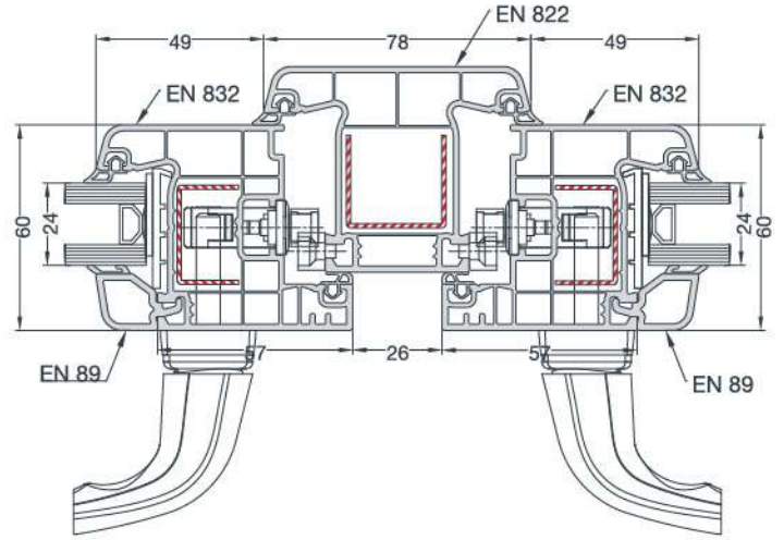
MULLION - WINDOW SASH INSTALLATION ORTA KAYIT - PENCERE KANAT UYGULAMASI
