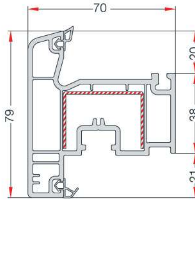
OUTWARD OPENING WINDOW SASH PROFILE DIŞA AÇILIM PENCERE KANAT PROFİLİ EN 23
