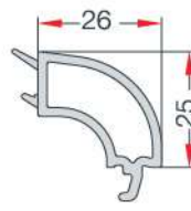
32-mm TRIPLE GLAZING BEAD 32 mm ÜÇLÜ CAM ÇİTASI EN 78
