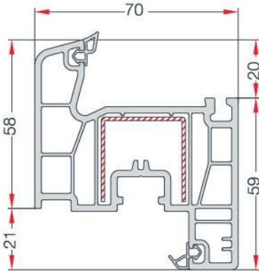
FRAME PROFILE KASA PROFİLİ EN 16
