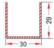
- U-SAC ORTA KAYIT
