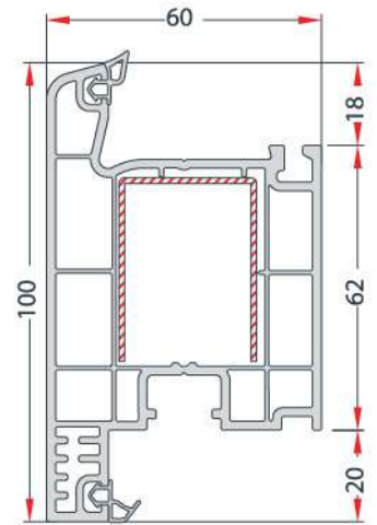
OUTWARD OPENING DOOR SASH PROFILE DIŞA AÇILIM KAPI KANAT PROFİLİ EN 88
