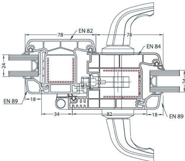
MULLION - DOOR SASH INSTALLATION ORTA KAYIT - KAPI KANAT UYGULAMASI
