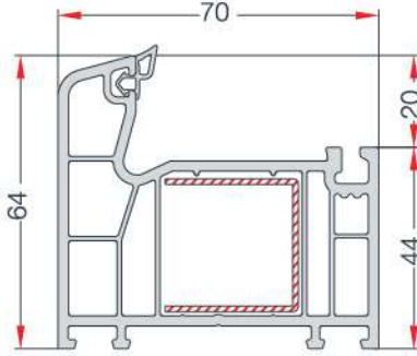
FRAME PROFILE KASA PROFİLİ EN 162
