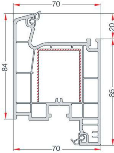
DOOR SASH PROFILE KAPI KANAT PROFİLİ EN 105
