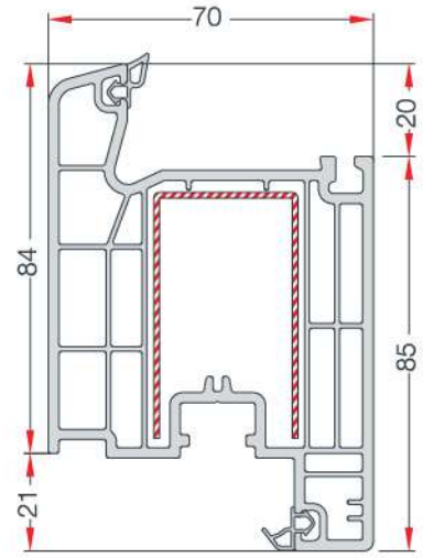
DOOR SASH PROFILE KAPI KANAT PROFİLİ EN 21
