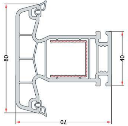
MULLION PROFILE ORTA KAYIT PROFİLİ EN 17
