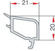
24-mm DOUBLE GLAZING BEAD 24 mm ÇİFT CAM ÇİTASI EN 49
