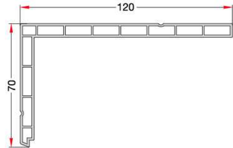
7 X 12 CASING PROFILE 7 x 12 PERVAZ PROFİLİ EN 51
