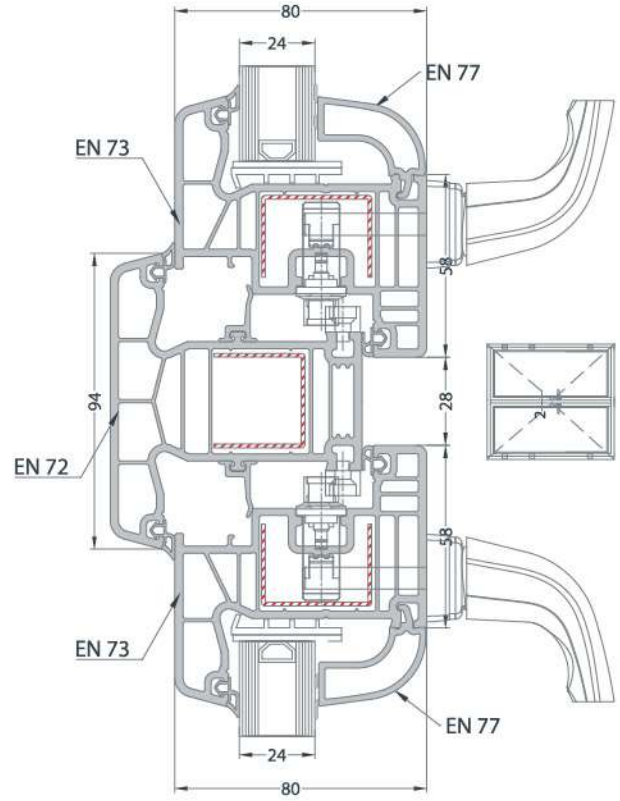
MULLION - WINDOW SASH INSTALLATION ORTA KAYIT - PENCERE KANAT UYGULAMASI
