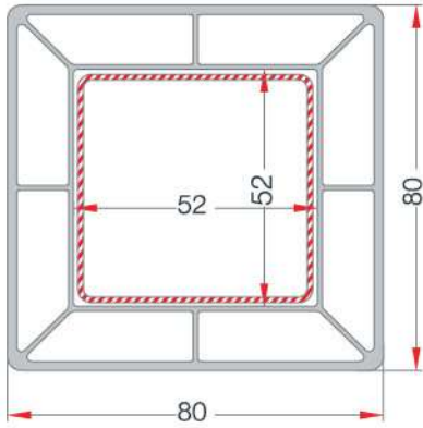
80x80 BOX PROFILE 80x80 KUTU PROFİLİ EN 27
