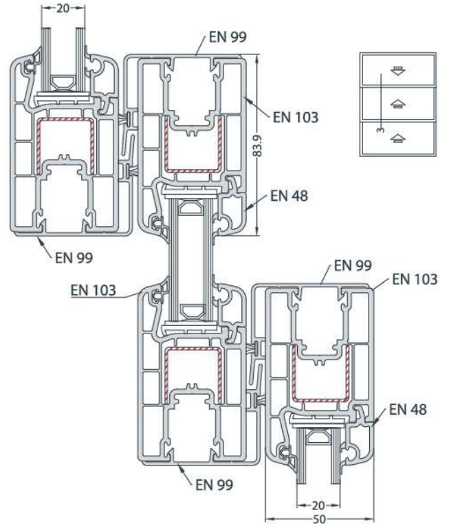
SLIDING LOCK ADAPTER INSTALLATION SÜRME KİLİT ADAPTÖR UYGULAMASI
