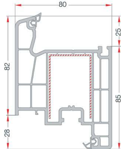
DOOR SASH PROFILE KAPI KANAT PROFİLİ EN 741
