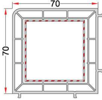
70x70 BOX PROFILE 70x70 KUTU PROFİLİ EN 55
