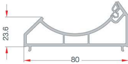
HIGHLINE CORNER ADAPTER HIGHLINE KÖŞE DÖNÜŞ ADAPTÖRÜ EN 29
