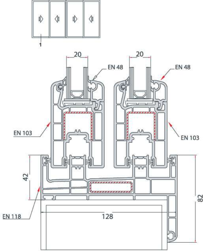
SLIDE WELL SLIDING FRAME - SLIDING SASH INSTALLATION SLIDE WELL SÜRME KASA - SÜRME KANAT UYGULAMASI
