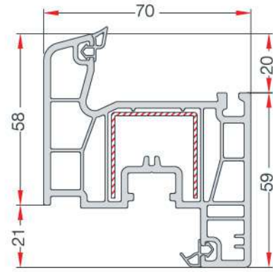
WINDOW SASH PROFILE PENCERE KANAT PROFİLİ EN 182
