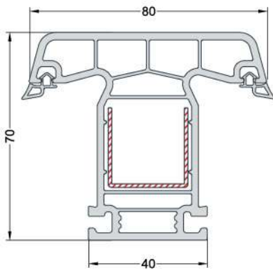
MULLION PROFILE ORTA KAYIT PROFİLİ EN 172
