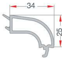
24-mm DOUBLE GLAZING BEAD 24 mm ÇİFT CAM ÇİTASI EN 77
