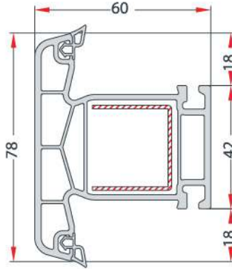
MULLION PROFILE ORTA KAYIT PROFİLİ EN 82
