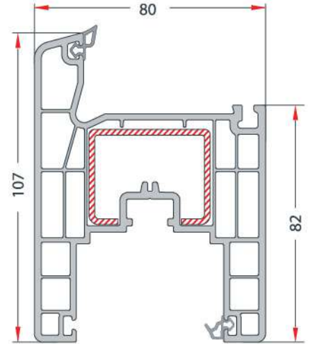
MASTERLINE SLIDING SASH PROFILE MASTERLINE SÜRME KANAT PROFİLİ EN 343
