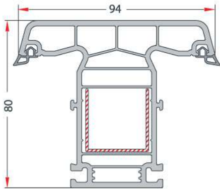
MULLION PROFILE ORTA KAYIT PROFİLİ EN 72
