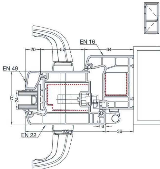
FRAME - OUTWARD OPENING DOOR SASH INSTALLATION KASA - DIŞA AÇILIM KAPI KANAT UYGULAMASI
