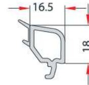
24-mm DOUBLE GLAZING BEAD 24 mm ÇİFT CAM ÇİTASI EN 89
