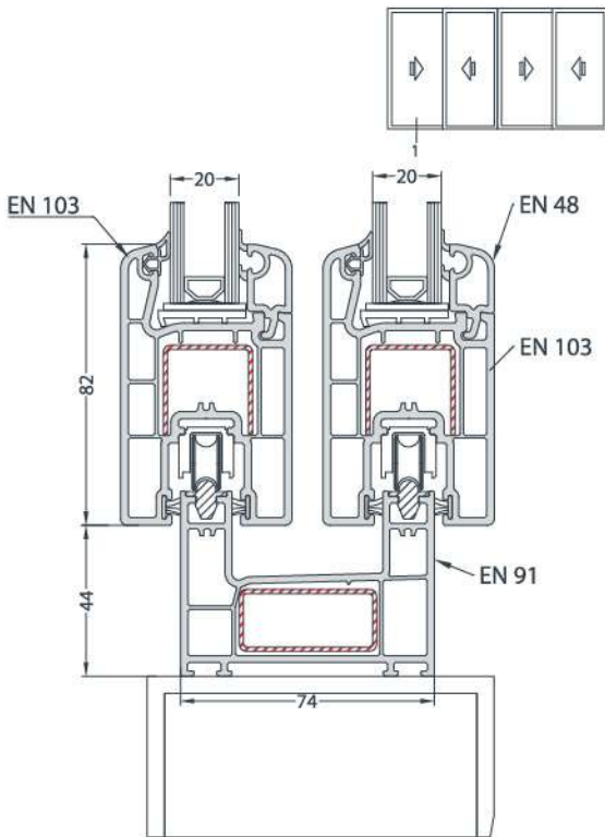
DOUBLE RAILED SLIDING FRAME - SLIDING SASH INSTALLATION SÜRME ÇİFT RAYLI KASA - SÜRME KANAT UYGULAMASI
