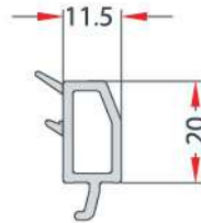
36-mm TRIPLE GLAZING BEAD 36 mm ÜÇLÜ CAM ÇİTASI EN 116
