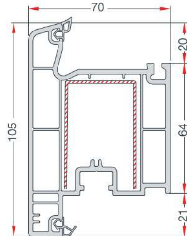
OUTWARD OPENING DOOR SASH PROFILE DIŞA AÇILIM KAPI KANAT PROFİLİ EN 22
