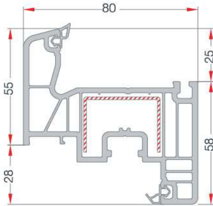
WINDOW SASH PROFILE PENCERE KANAT PROFİLİ EN 73
