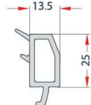
44-mm TRIPLE GLAZING BEAD 44 mm ÜÇLÜ CAM ÇİTASI EN 117
