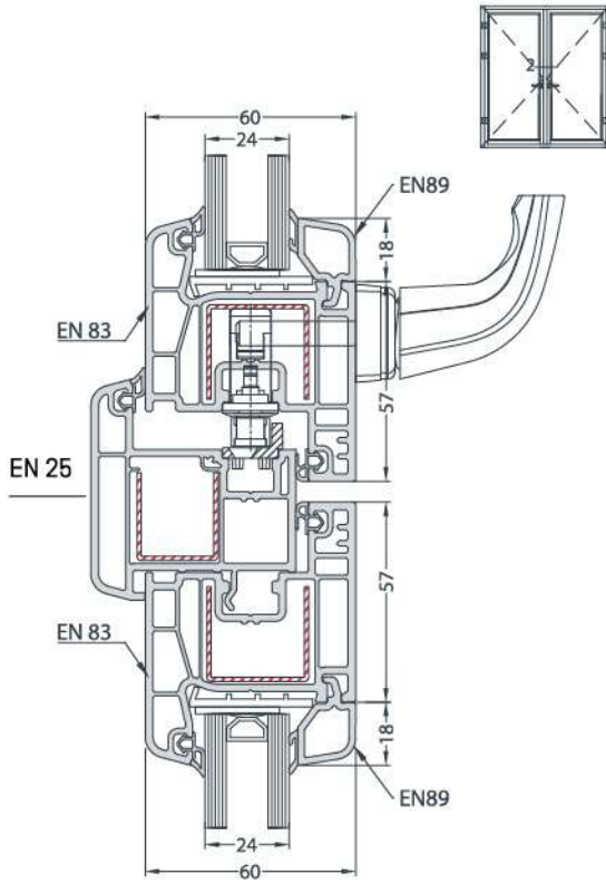
MOVABLE MULLION - WINDOW SASH INSTALLATION HAREKETLİ ORTA KAYIT - PENCERE KANAT UYGULAMASI
