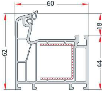
FRAME PROFILE KASA PROFİLİ EN 81
