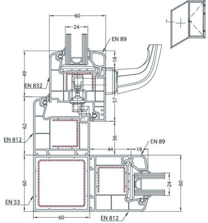
BOX PROFILE INSTALLATION KUTU PROFİLİ UYGULAMASI
