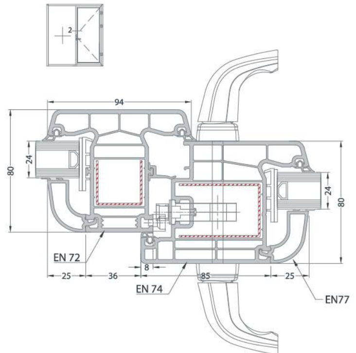
MULLION - DOOR SASH INSTALLATION ORTA KAYIT - KAPI KANAT UYGULAMASI
