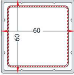
60x60 BOX PROFILE 60x60 KUTU PROFİLİ EN 53
