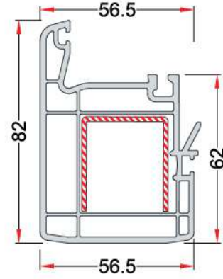
VERTICAL SLIDING MULLION PROFILE DİKEY SÜRME ORTA KAYIT PROFİLİ EN 97
