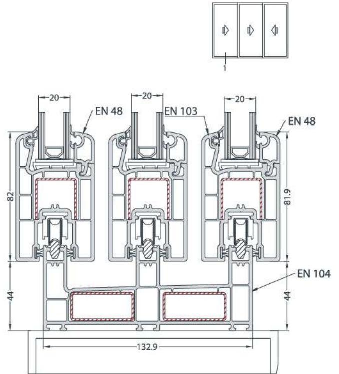
TRIPLE RAILED SLIDING FRAME - SLIDING SASH INSTALLATION SÜRME 3 RAYLI KASA - SÜRME KANAT UYGULAMASI
