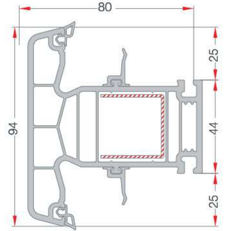
MULLION PROFILE ORTA KAYIT PROFİLİ EN 72
