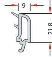
24-mm DOUBLE GLAZING BEAD 24 mm ÇİFT CAM ÇİTASI EN 109
