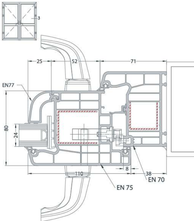
FRAME - OUTWARD OPENING DOOR SASH INSTALLATION KASA - DIŞA AÇILIM KAPI KANAT UYGULAMASI
