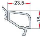
18-mm DOUBLE GLAZING BEAD 18 mm ÇİFT CAM ÇITASI EN 41
